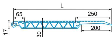
Profil de fermeture latéral (proposé en option)
