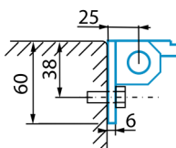
Détail charnière
