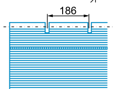
Détail charnière repère 3
